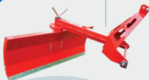
Série MINILIV de lames de nivelage pour mini-tracteur Largeur de travail de 90 à 140 cm
