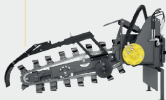
CTM 120 trancheuse pour tracteur Pour prise de force (PDF) de tracteur Profondeur de tranchée 120 cm
