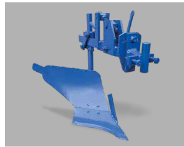
CHARRUE SIMPLE
